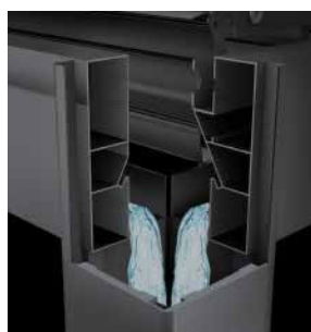
Évacuation de l'eau par les poteaux verticaux
